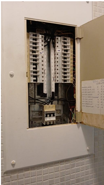
IMAGEM 38: Disjuntores sem a placa de proteção.
