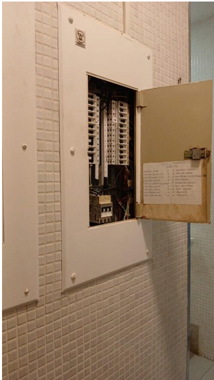
IMAGEM 39: Os quadros de disjuntores sempre deverão ter fixado na porta pela parte de dentro a identificação de cada disjuntor.
